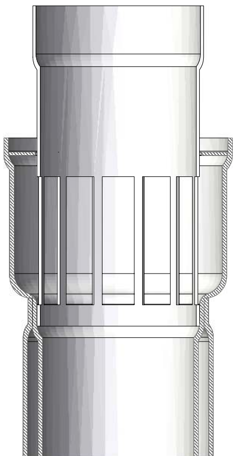
Vesiset Plus siivilämuhvi kerroksiin ilman palokatkonauhaa.
